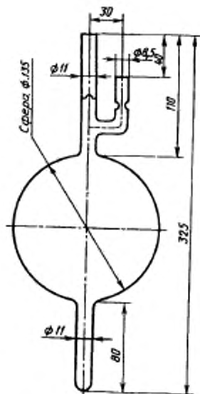
Черт. 13
