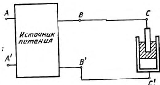
Схема электропитания печи
