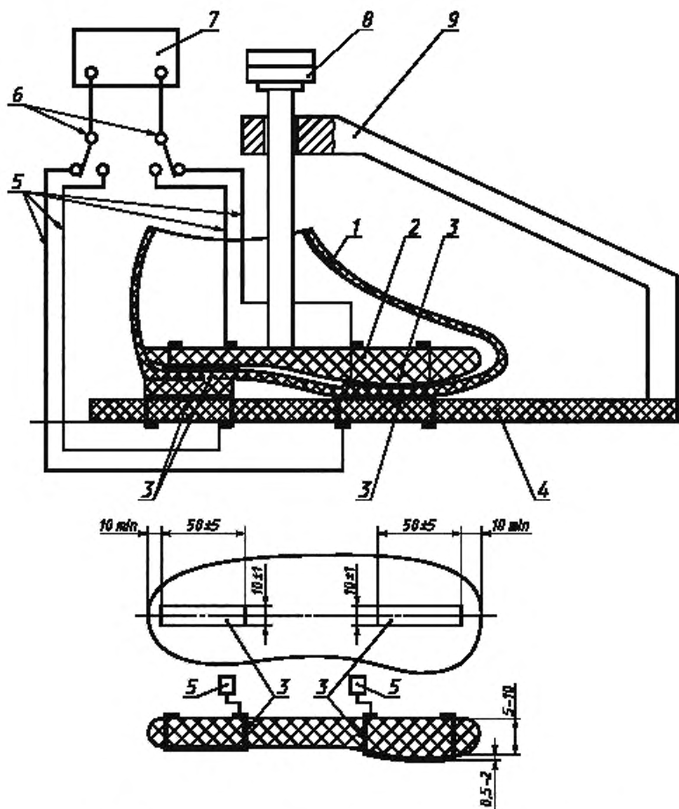
1 — специальная обувь; 2 — колодка (стелька) пластмассовая; 3 — электроды; 4 — пластмассовая пластина; 5 — провода; 6 — переключатель; 7 — измерительный прибор; 8 — груз; 9 — станина
