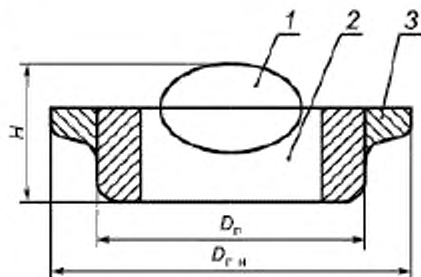
1 — запирающий элемент; 2 — проходное отверстие; 3 — фланец пришивного кольца, H — высота ПКС, D_г — посадочный диаметр ПКС; D_{г.н} — пришивной наружный диаметр ПКС
