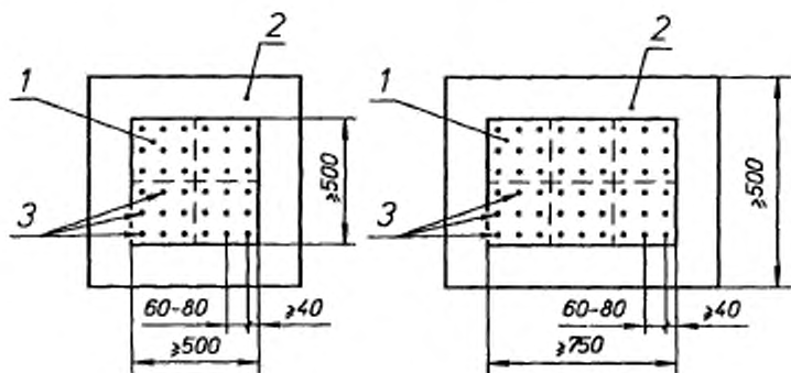
1 — испытательный участок; 2 — обрамляющий бортик; 3 — точки приложения ударов
