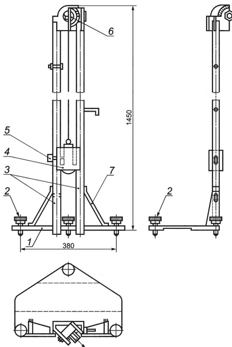
1 — площадка с прорезью для прохода гирь; 2 — регулировочные винты; 3 — вертикальные направляющие; 4 — гиря с боковыми пазами и бойком; 5 — выдвижные штоки; 6 — направляющий ролик; 7 — подкосы
