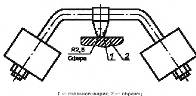
Рисунок 14 — Установка для испытания прочности материалов при нагревании
