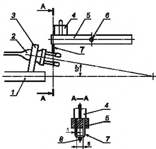
1 — основание; 2 — образец; 3 — зажим; 4 — груз; 5 — стержень; 6 — ось; 7 — стальная проволока; 8 — штырь вилок
