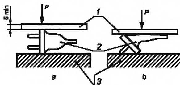
Р — усилие 150 Н; 1 — стальная нажимная пластина; 2 — образец; 3 — стальное основание
