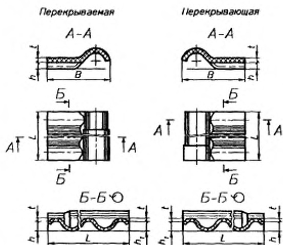
Рисунок 2 — Коньковые детали
