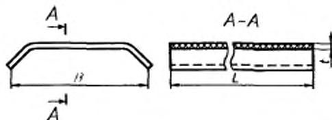
Рисунок 5 — Лотковая деталь
