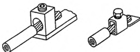
Контактный зажим с прямым прижатием жилы проводника
