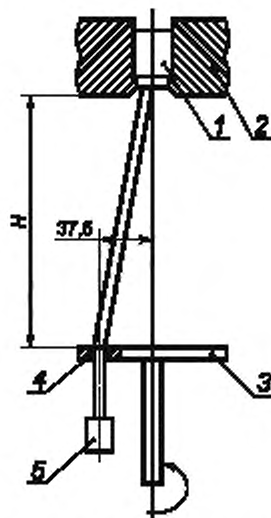
1 — зажим; 2 — подставка; 3 — плита; 4 — втулка; 5 — груз
