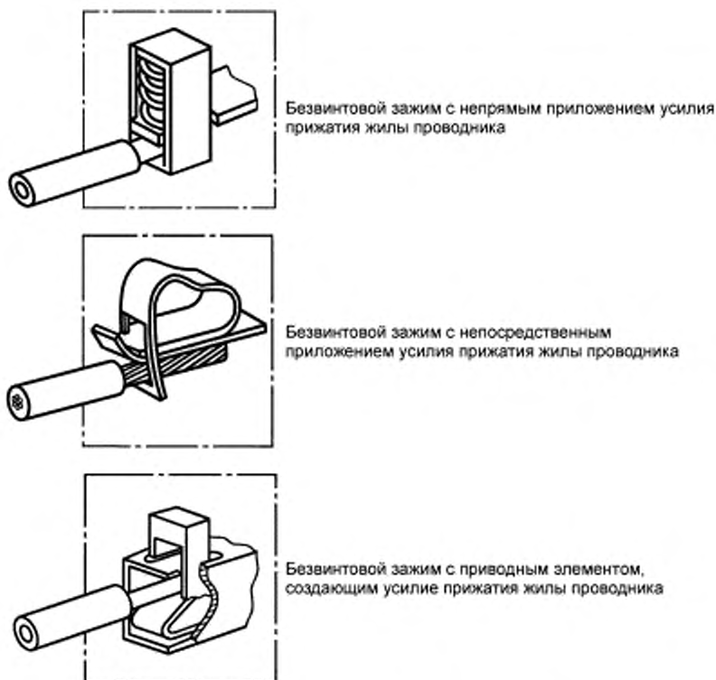
Рисунок 6 — Примеры безвинтовых контактных зажимов
