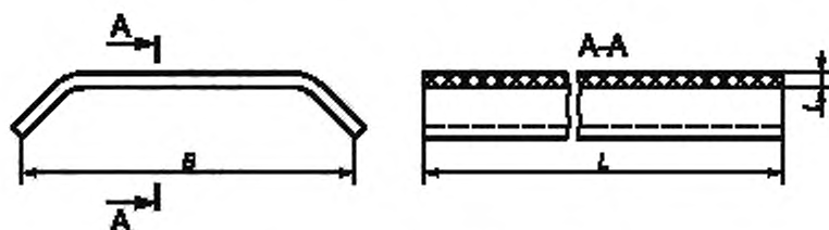
Рисунок 10 — Лотковая деталь
