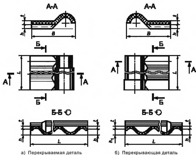
Рисунок 6 — Коньковые детали
