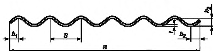
Рисунок 4 — Профиль листа 40/150 с симметричными кромками
