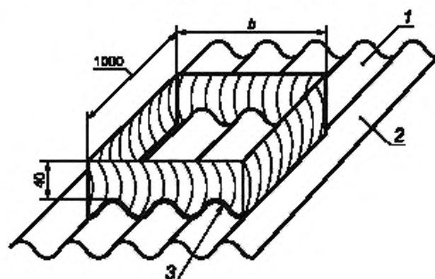
Рисунок 23 — Рама для определения водонепроницаемости
