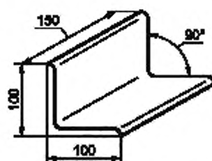
Рисунок 12 — Металлический упор для измерения длины и ширины
