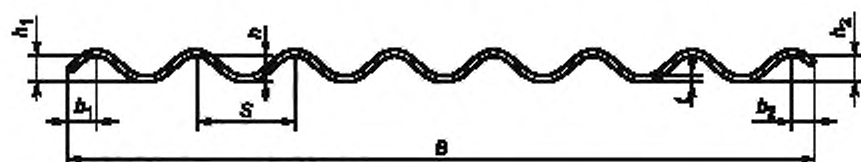
Рисунок 4 — Профиль листа 40/150 с симметричными кромками
