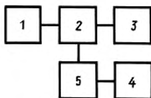
1 — проверяемый радиопередатчик; 2 — устройство связи; 3 — эквивалентное нагрузочное сопротивление (эквивалент антенны); 4 — электронно-счетный частотомер; 5 — аттенюатор
