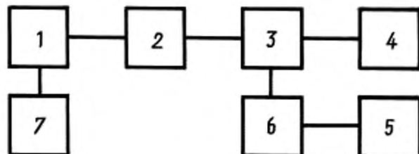
Рисунок 5 — Структурная схема измерения частоты радиопередатчиков с излучением класса J3E
