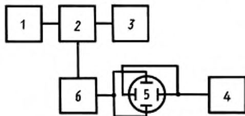
1 — проверяемый радиопередатчик; 2 — устройство связи; 3 — эквивалентное нагрузочное сопротивление (эквивалент антенны); 4 — генератор образцовой частоты; 5 — осциллограф; 6 — аттенюатор
