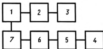
1 — опорный генератор радиопередатчика; 2 — проверяемый радиопередатчик; 3 — эквивалентное нагрузочное сопротивление (эквивалент антенны); 4 — стандарт частоты; 5 — компаратор частоты; 6 — аттенюатор; 7 — устройство связи.
