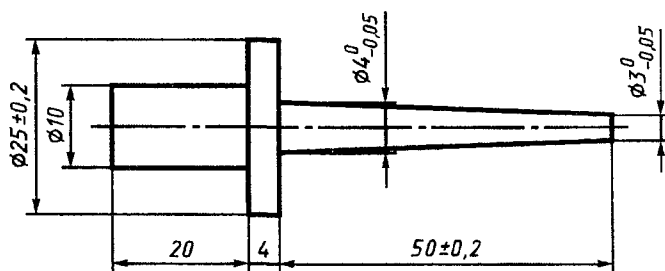
Рисунок 101 — Длинный испытательный стержень
