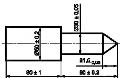
Рисунок 3 – Испытуемый шуп
