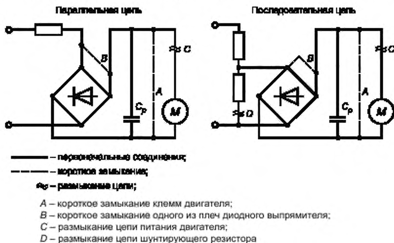
Рисунок F.1 – Имитация неисправностей
