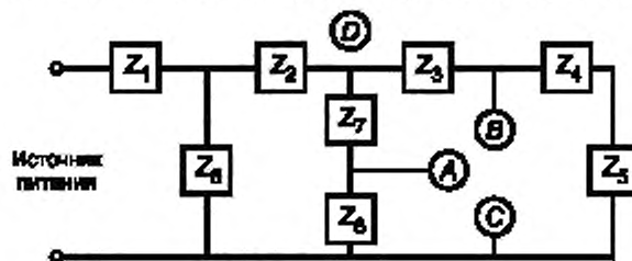
D – наиболее удаленная от источника питания точка, в которой мощность, подаваемая на внешнюю нагрузку, превышает 15 Вт A и B – наиболее близкие к источнику питания точки, в которых мощность, подаваемая на внешнюю нагрузку, не превышает 15 Вт. Это маломощные точки. Точки A и B раздельно накоротко соединены с точкой C . Условия повреждения а) – г) по 20.11.2 рассматриваются в каждой из цепей Z_1 , Z_2 , Z_3 , Z_5 и Z_7 при необходимости
