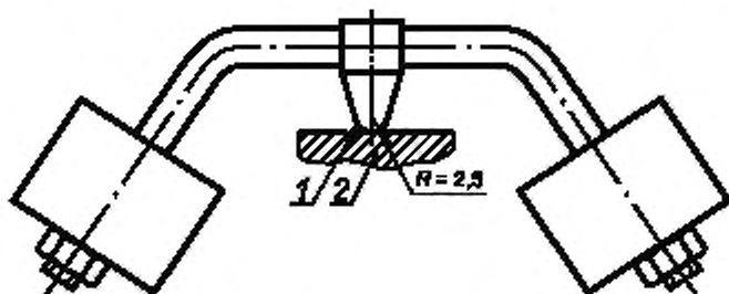
Рисунок 12 – Устройство для вдавливания шарика
