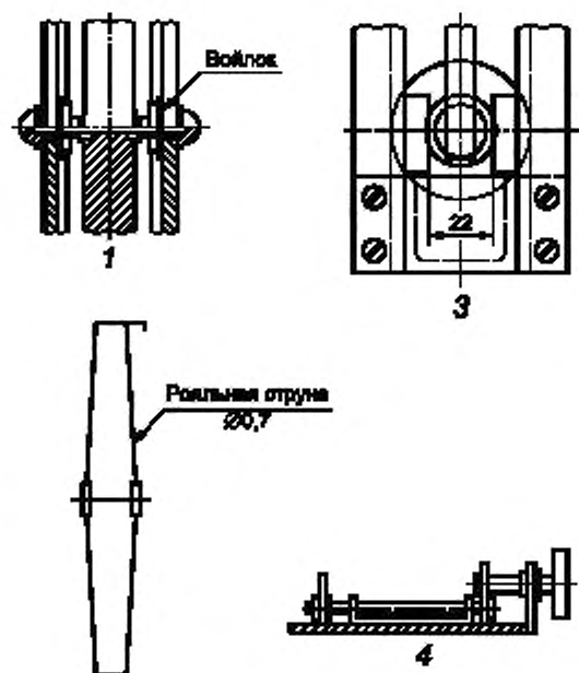
Рисунок R.5 – Детали калибрующего устройства
