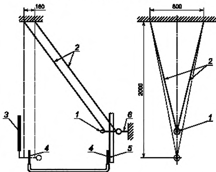
Рисунок R.6 – Установка для настройки калибрующего устройства
