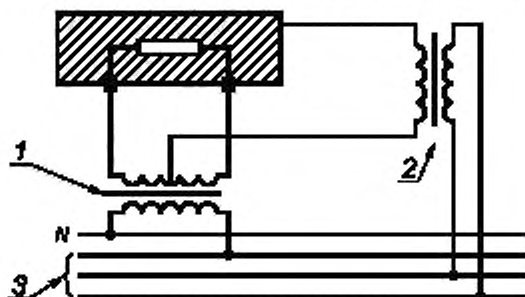
1 – разделительный трансформатор; 2 – повышающий трансформатор; 3 – трехфазная сеть
