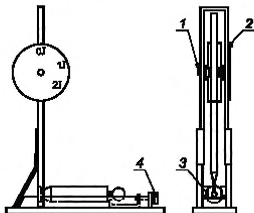
1 - подшипник; 2 - фиксирующий указатель; 3 - спусковое основание; 4 - спусковой механизм
