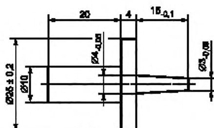
Рисунок 2 – Испытуемый стержень
