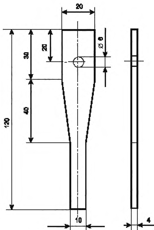
Рисунок R.3 – Стальная пружина
