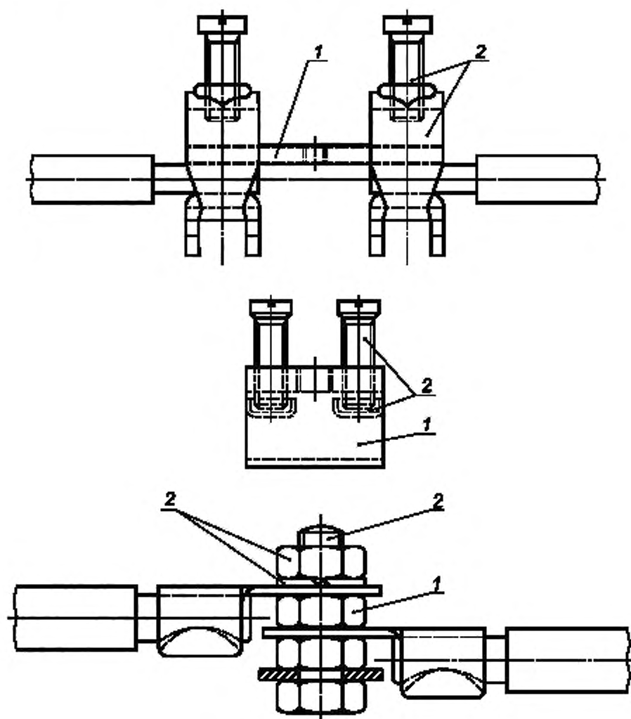
Рисунок 14 – Примеры частей заземляющих зажимов
