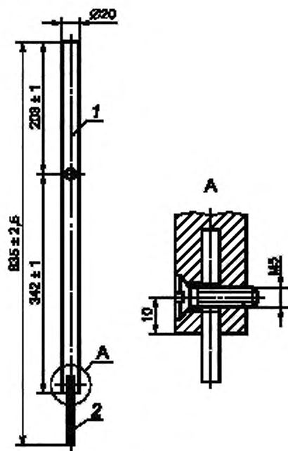
Рисунок R.2 – Маятник
