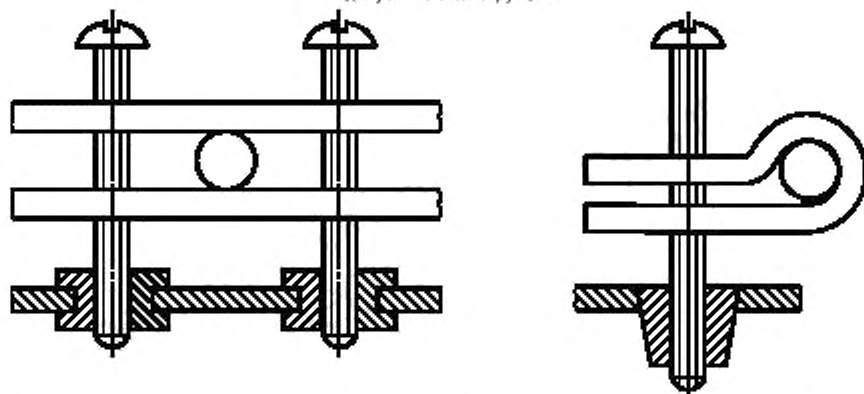
Рисунок 13 – Примеры выполнения крепления шнура
