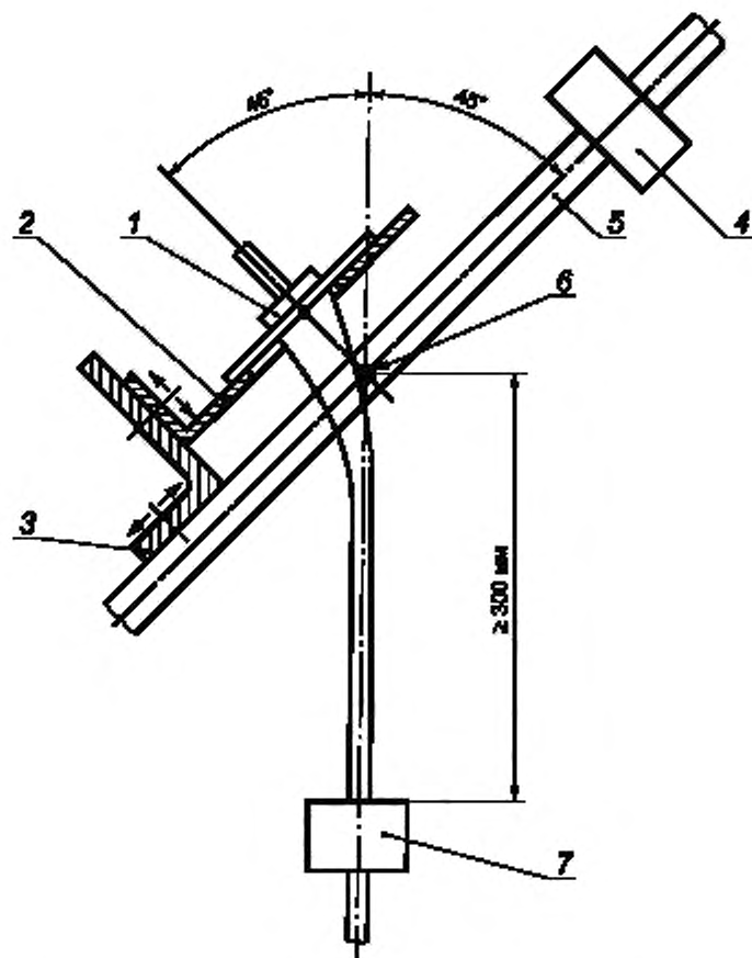
1 – образец; 2 – регулируемая несущая плата; 3 – регулируемый хронштейн; 4 – противовес, 5 – качающаяся рама; 6 – ось качения; 7 – груз
