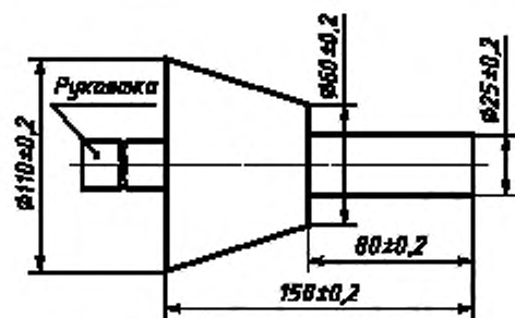
Рисунок 101 — Испытательный калибр
