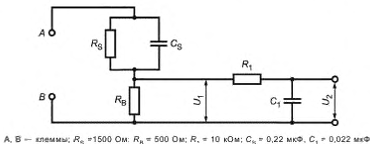
Рисунок D.1 — Измерительный прибор
