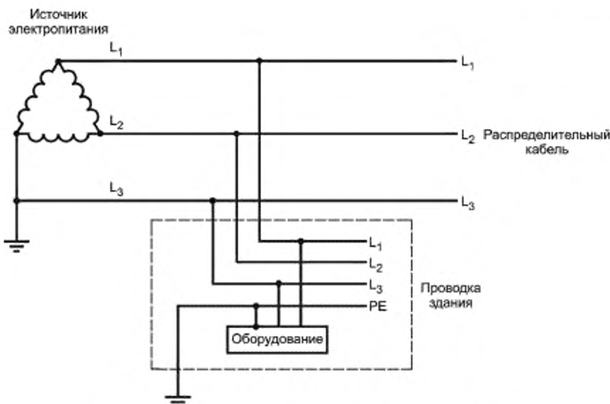
Рисунок V.6 — Пример TT-системы электропитания с тремя фазами
