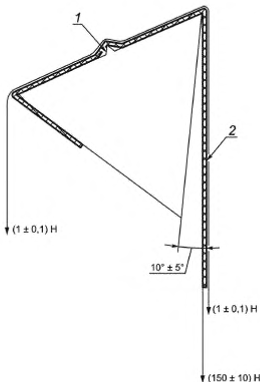
1 — шип; 2 — металлическая фольга
