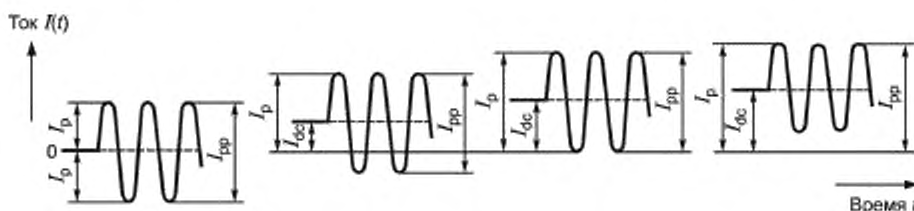
Рисунок М.3 — Двойная амплитуда тока и пиковое значение тока относительно земли
