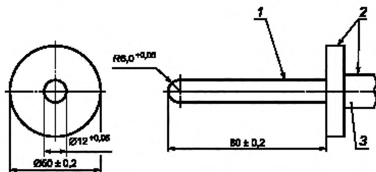
Рисунок 2С — Испытательный шуп
