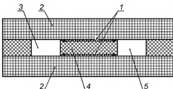
Рисунок F.15 — Тонколистовой изоляционный материал
