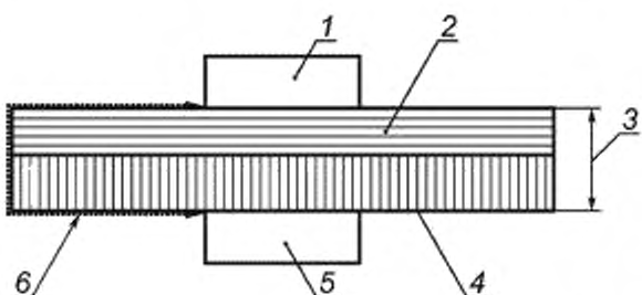
1 — проводящая часть 1, 2 — слой изоляции 1; 3 — требования к минимальному расстоянию через изоляцию нет, 4 — слой изоляции 2; 5 — проводящая часть 2, 6 — зазор и путь утечки (равны)
