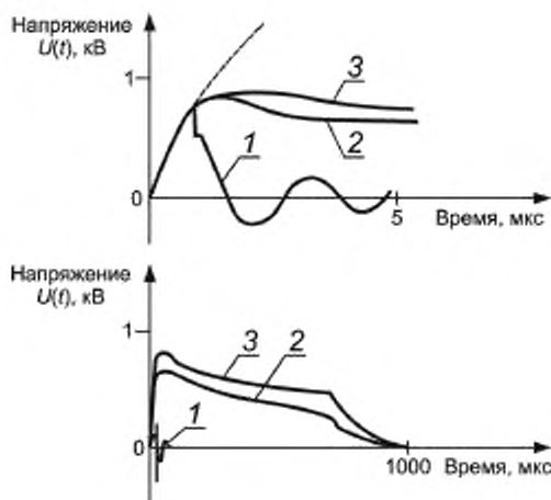
Тип ограничителя перенапряжений 1 — газоразрядный; 2 — полупроводниковый; 3 — металлооксидный
