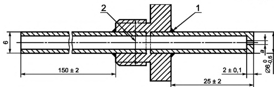
1 — резьба G1/4 А по [2]; 2 — пайка серебром
