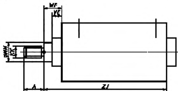
Рисунок 1 — Основные размеры
