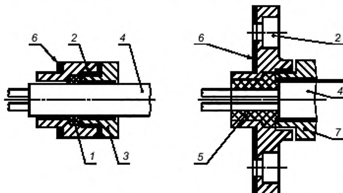
1 — уплотнительное кольцо; 2 — корпус ввода; 3 — нажимная деталь; 4 — кабель; 5 — заливочный компаунд; 6 — уплотнение; 7 — деталь, фиксирующая компаунд
