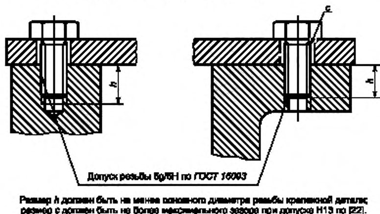
Рисунок 1 — Допуски и зазор для резьбовых крепежных деталей
