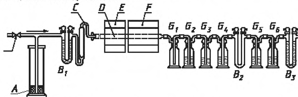
Рисунок 1 — Установка для сжигания и абсорбции
