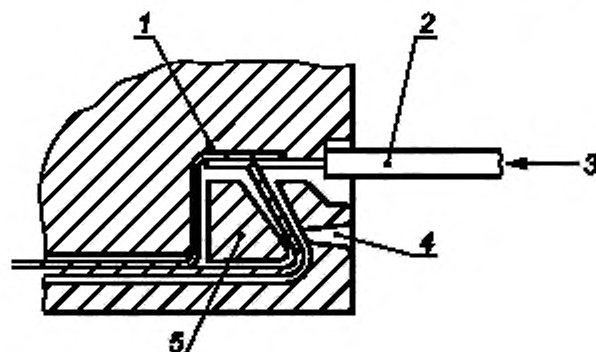
1 — токоведущий проводник; 2 — для испытания растягивающим усилием 15 Н; 3 — проводник, рассчитанный на максимальный ток 3 А; 4 — устройство разъединения; 5 — ограничитель
