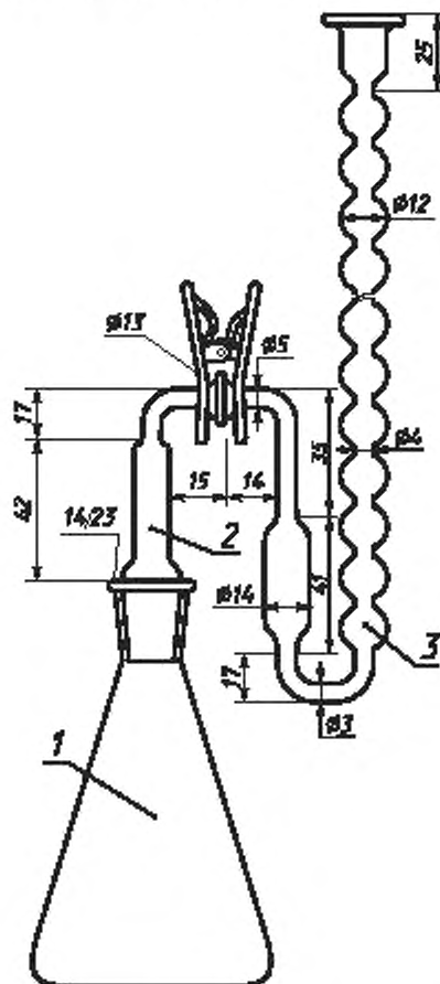
1 — коническая колба; 2 — соединительная трубка; 3 — абсорбер
