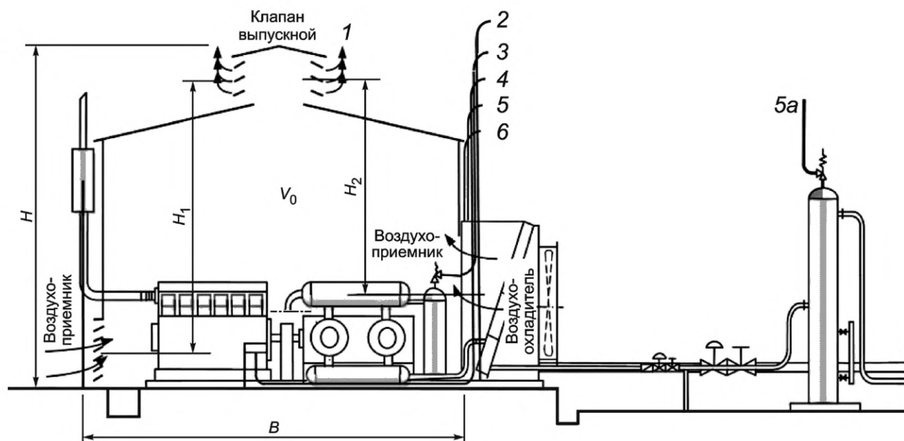
1 — вентиляционный проем для выхода воздуха; 2 — пусковой клапан газа; 3 — клапан продувки компрессора; 4 — запорный клапан топливного газа; 5 и 5a — клапаны сброса давления; 6 — клапан сальника поршневого штока
