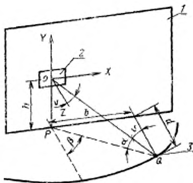
1 — наружная стена; 2 — испытываемый образец; 3 — громкоговоритель
