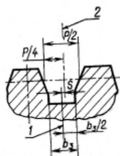
Положение оси симметрии канавки: 1 — действительное, 2 — номинальное
