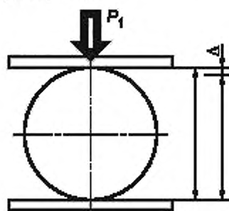
Рисунок 2 — Схема испытания модельных образцов гипсовых повязок цилиндрической формы для определения величины остаточной деформации при диаметральной сжатии
