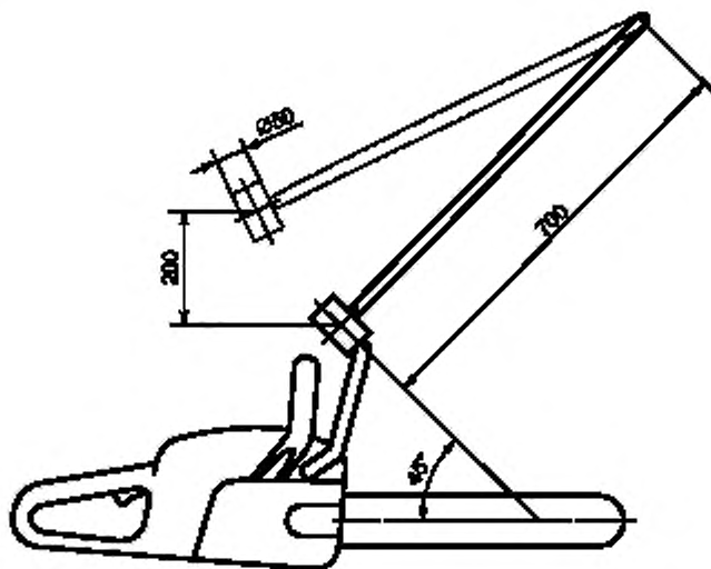
Рисунок 1 — Маятниковая система
