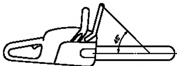
Рисунок 2 — Статическое испытание на усилие срабатывания тормоза
