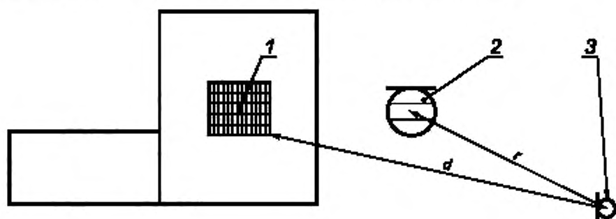
1 — доминирующий источник шума машины; 2 — положение образцового источника шума; 3 — микрофон
