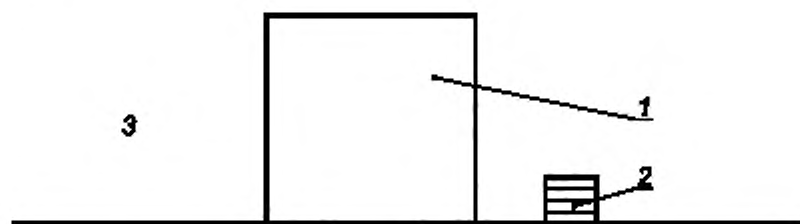
1 — машина как экран; 2 — положение образцового источника шума; 3 — область экранирования, когда работает образцовый источник шума (при выключенной машине). Один микрофон помещают в этой области
