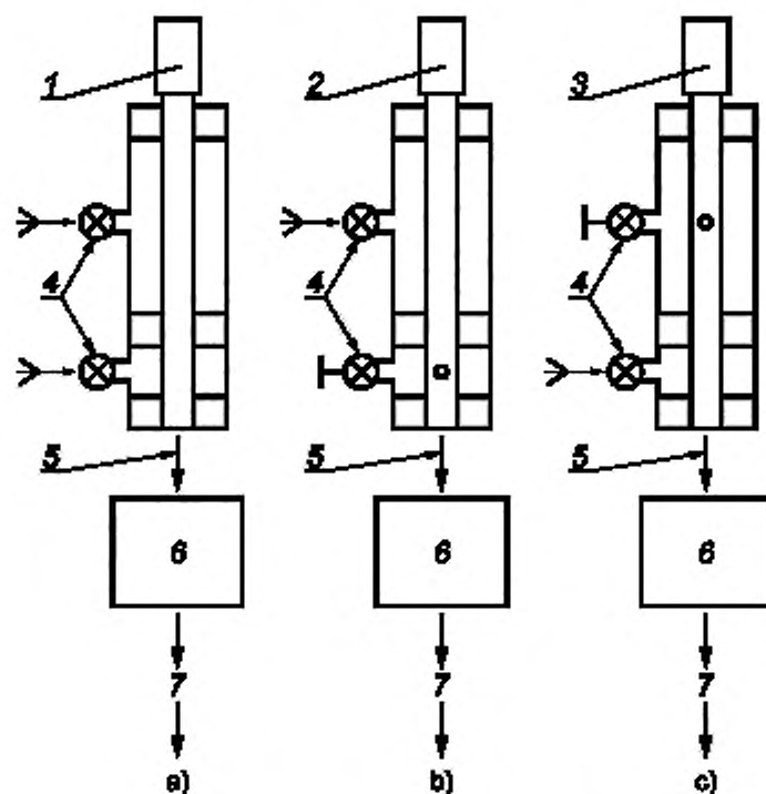
1 — насадка перепада давления (вставлен калибр перепада давления); 2 — насадка для тестирования утечек вентиляционной камеры фильтра; 3 — насадка для тестирования утечек вентиляционной камеры сигаретного штранга; 4 — изоляционные клапаны вентиляционных камер; 5 — перепад давления; 6 — устройство для измерения объемного потока, 7 — общий поток пропускаемого воздуха
