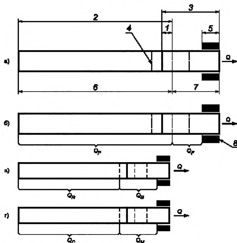
1 — перекрытие ободковой бумагой отрезка сигаретного штранга; 2 — сигаретная бумага; 3 — ободковая бумага; 4 — отметка длины окурка; 5 — стандартная глубина вставки сигареты ГОСТ ISO 3308; 6 — сигаретный штранг; 7 — фильтр; 8 — устройство для вставки сигарет (держатель для сигарет); Q — общий поток воздуха; Q_F — вентиляционный поток фильтра; Q_P — вентиляционный поток сигаретного штранга; Q_B — вентиляционный поток окурка; Q_M — вентиляционный поток сжигаемой части сигаретного штранга; Q_C — вентиляционный поток ободковой бумаги; Q_C — вентиляционный поток сигаретной бумаги
