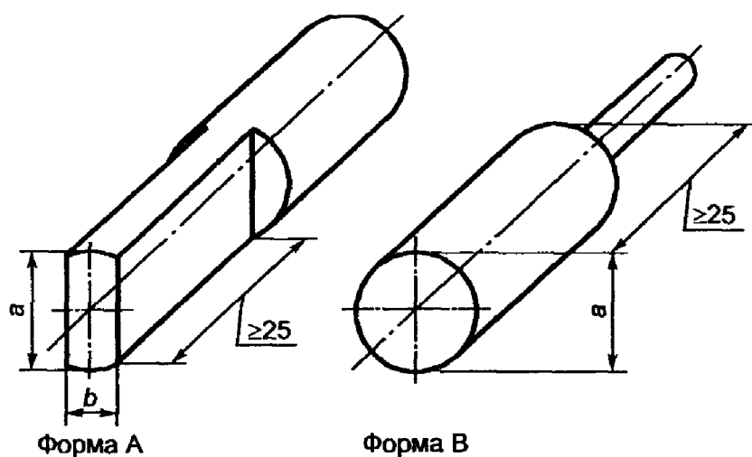
Рисунок 5 - Щупы (см. 9.2.4.5)
