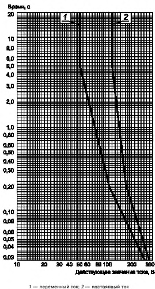
Рисунок С.1 — Кривая продолжительности предполагаемого напряжения прикосновения в соответствии с таблицей С.1
