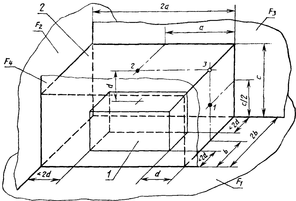
1—огнибающий параллелепипед отсчета; 2—измерительная поверхность; F_1, \dots, F_4 —звукоотражающие поверхности; ● —основные точки измерения 1 и 2; ○ —дополнительная точка измерения 3
