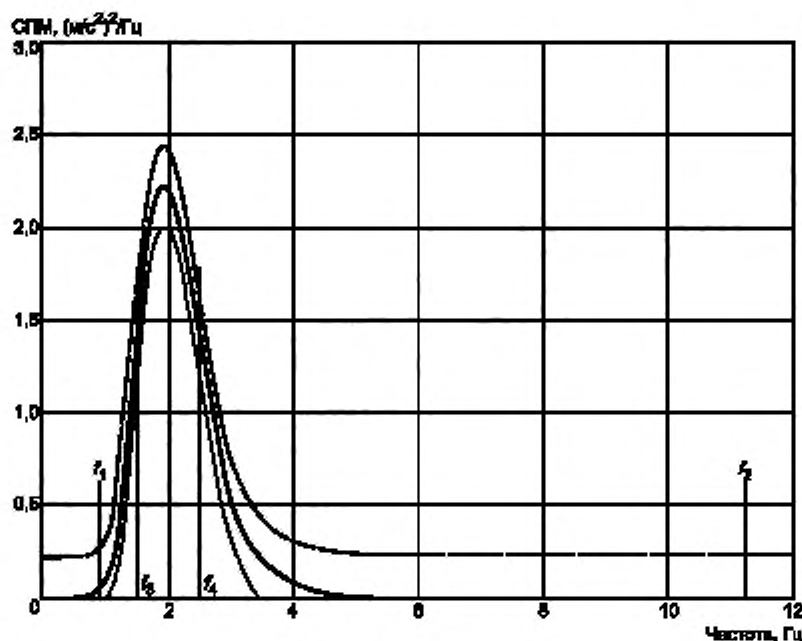
Рисунок 2 — СМ для спектрального класса ЕМ 1 (самосвал с жесткой или шарнирно-сочлененной рамой снаряженной массой более 4500 кг)
