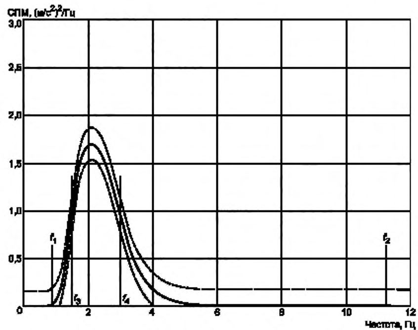
Рисунок 4 — СПМ для спектрального класса ЕМ 3 (колесные погрузчики массой более 4500 кг)
