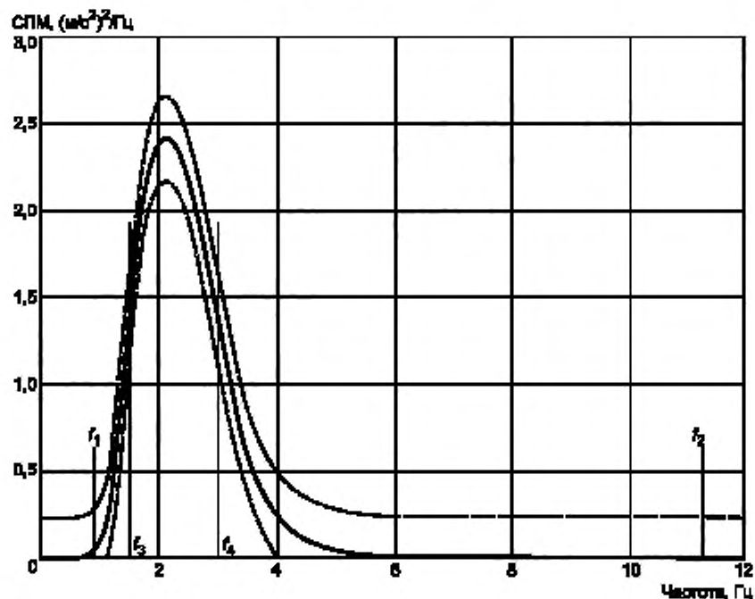
Рисунок 3 — СПМ для спектрального класса ЕМ 2 (скрепер без подвески мостов или рамы)
