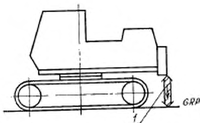
I — стальная линейка
