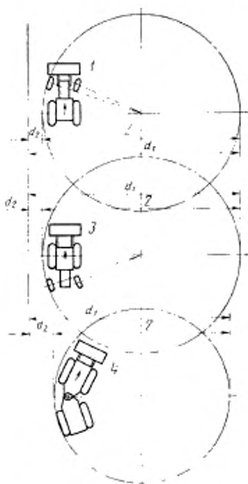
Ширина полосы безостановочного разворота
