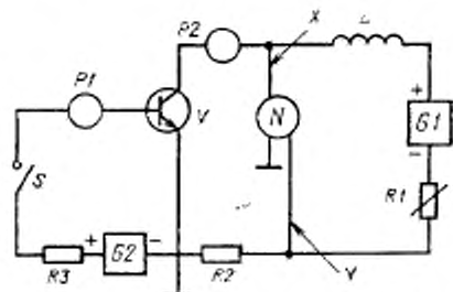
P1, P2 — измерители постоянного тока; G1 — источник напряжения; G2 — источник тока; R1, R2, R3 — резисторы ( R2 — безиндуктивный измерительный); L — индуктивность; S — переключатель; N — осциллоскоп; V — испытуемый транзистор
