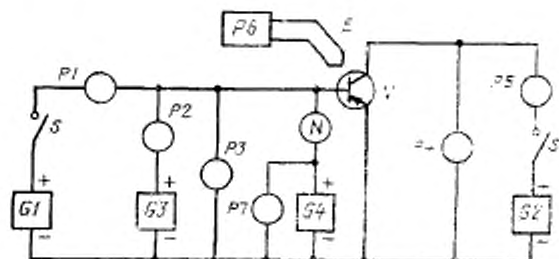
P1, P2, P5 — измерители постоянного тока; P3, P7, P4 — измерители постоянного напряжения; S — электроинный или электромеханический ключ; G3 — регулируемый источник стабилизированного постоянного тока; G4 — регулируемый источник стабилизированного постоянного напряжения; G1, G2 — источники постоянного тока. N — осциллоскоп для регистрации изменения температуры во времени; P6 — потенциометр постоянного тока; E — термодара (или другое устройство для измерения температуры бор-уса). V — испытуемый транзистор
