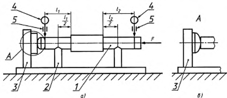
1 — образец-изделие типа «валик»; 2 — призма; 3 — осевой упор; 4 — измерительный прибор; 5 — державка
