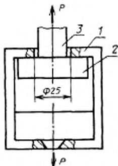
1—захват образца; 2—образец; 3—металлический цилиндр;
