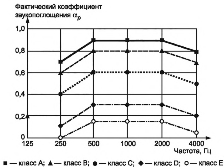
Рисунок В.1 — Нормативные кривые, ограничивающие классы звукопоглощения
