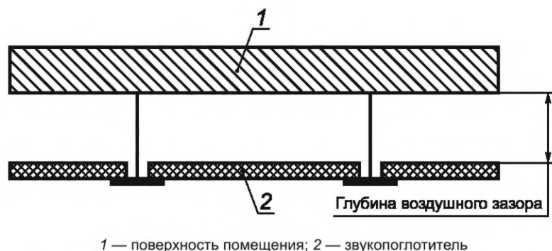
Рисунок 2 — Схема размещения образцов материала при проведении испытаний
