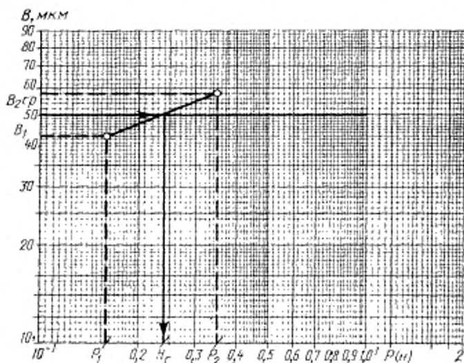
ДИАГРАММА ДЛЯ ОПРЕДЕЛЕНИЯ ТВЕРДОСТИ ЦАРАПАНИЕМ [ H_C ]
