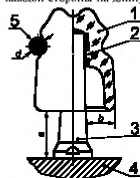
1 — изолятор; 2 — уплотнитель; 3 — штырь; 4 — траверса; 5 — проводник; а — расстояние от нижнего края юбки до траверсы; b — расстояние от края юбки до штыря; d — диаметр проводника
