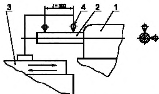
1 — задняя бабка; 2 — оправка; 3 — каретка; 4 — индикатор
