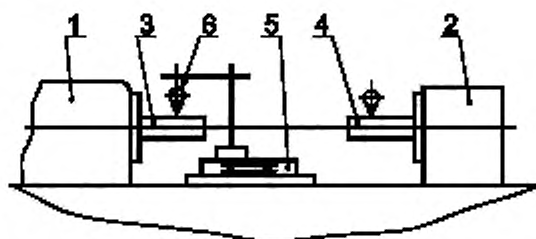
1 — передняя бабка; 2 — задняя бабка; 3, 4 — оправки; 5 — каретка; 6 — индикатор
