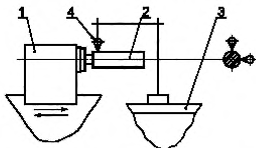
1 — шлифовальная бабка; 2 — контрольная втулка; 3 — станина изделия; 4 — индикатор
