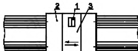
1 — уровень; 2 — каретка; 3 — шлифовальная бабка
