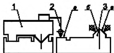
1 — каретка; 2 — индикатор; 3 — станина изделия
