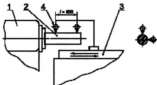
1 — передняя бабка; 2 — оправка; 3 — каретка; 4 — индикатор
