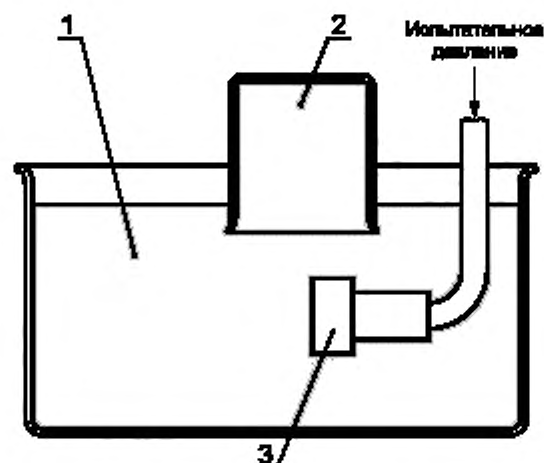
1 — сосуд, наполненный изопропиловым спиртом или другой соответствующей жидкостью; 2 — перевернутый мерный цилиндр для сбора пузырьков, наполненный жидкостью; 3 — испытуемое соединение
