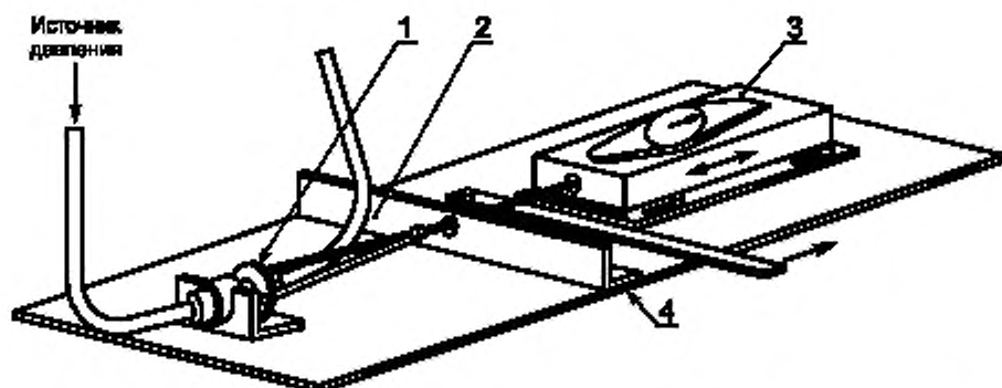
1 — устройство для присоединения динамометра к заправляющей втулке втычной части; 2 — защитная плита; 3 — динамометр; 4 — основание приспособления, показывающего, что функцию можно изменить, чтобы наилучшим образом приспособить к испытываемому соединению
