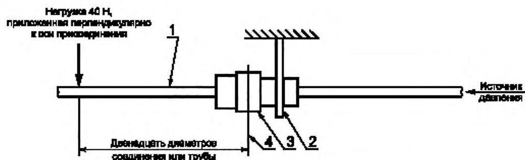
1 — стержень, присоединенный к части соединения, не закрепленной в приспособлении; 2 — приспособление для закрепления части соединения; 3 — испытуемое соединение; 4 — ось запорного устройства
