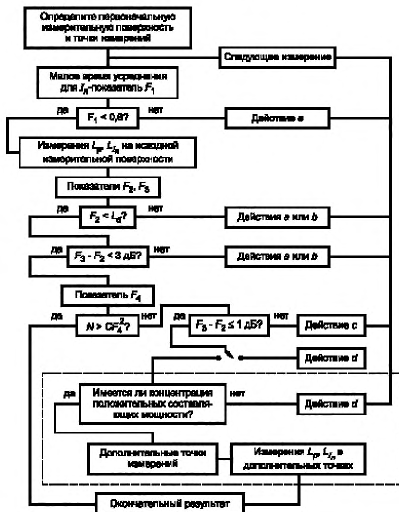
Рисунок Б.1 — Алгоритм достижения необходимой точности
