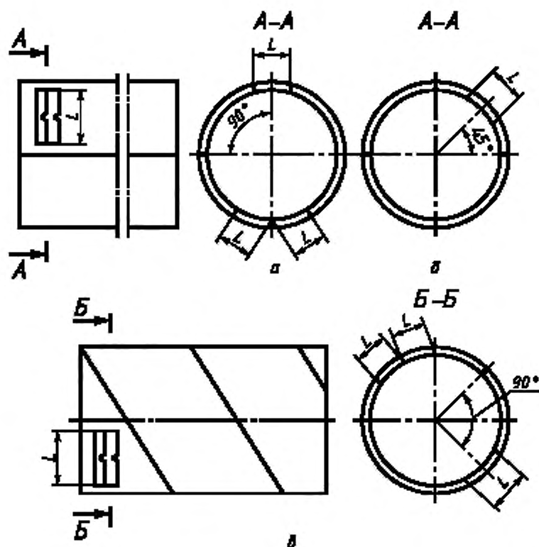
а — прямошовная труба с одним швом; б — прямошовная труба с двумя швами; в — спирально-шовная труба; L — длина образца
