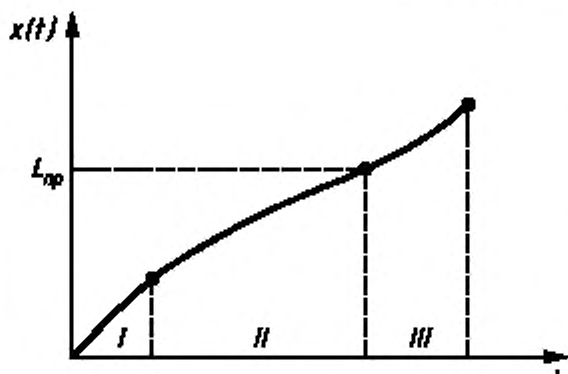
Рисунок 1 — Характер процесса изнашивания
