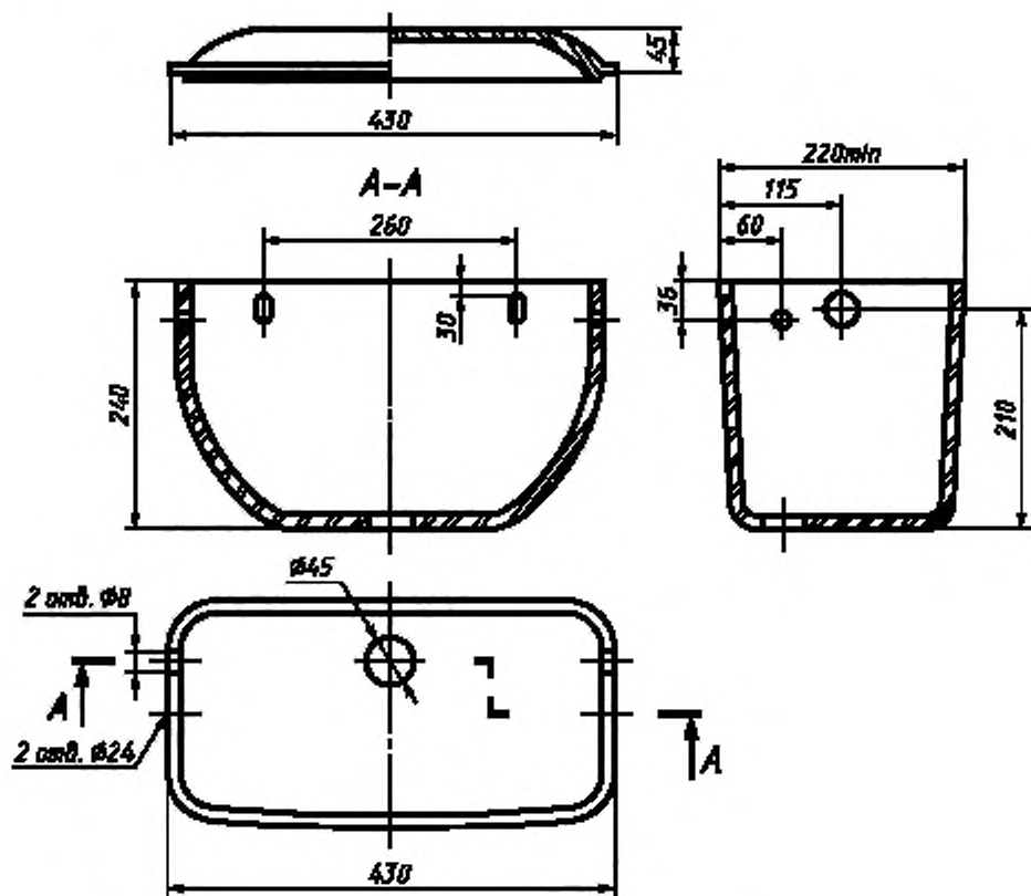
Рисунок 10 — Бачок смывной высокорасполагаемый с боковым пуском
