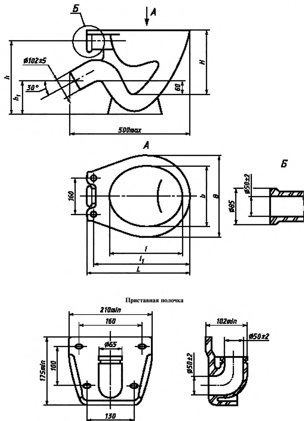
Рисунок 8 — Унитаз с приставной полочкой
