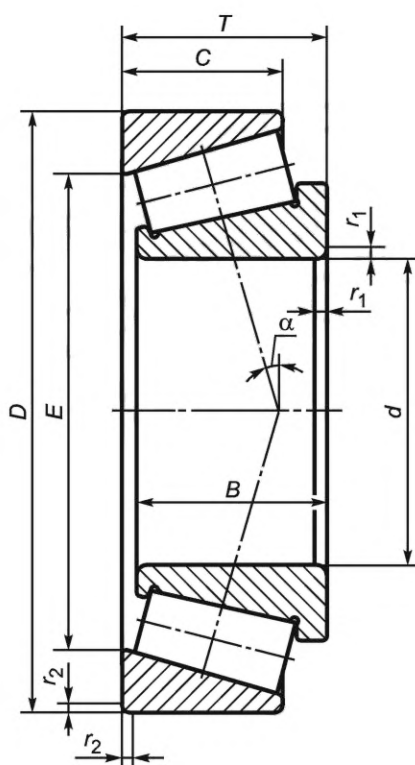
Рисунок 1 — Конструктивные исполнения 00, 02
