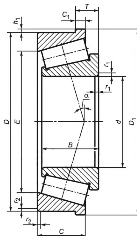
Рисунок 2 — Конструктивные исполнения 06, 62
