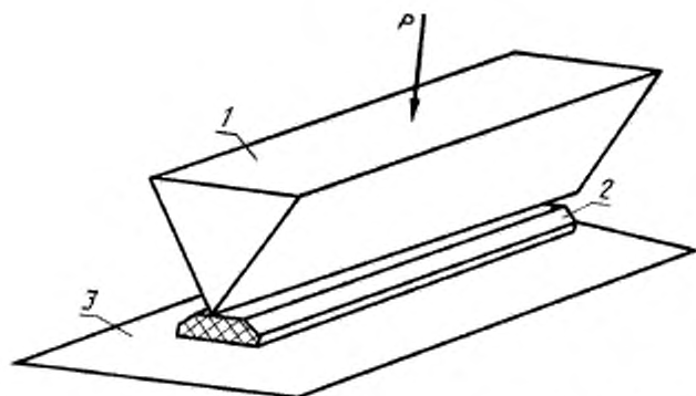
1—треугольная металлическая призма; 2—образец стеклопластика; 3—опорная плита
