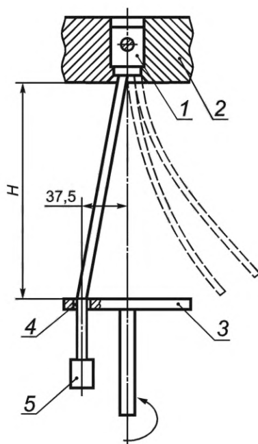
1 — зажим; 2 — подставка; 3 — плита; 4 — втулка; 5 — груз
