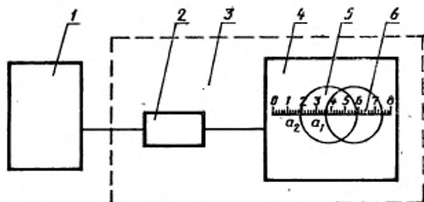
Схема контроля отклонения от соосности с использованием ПТУ-43
