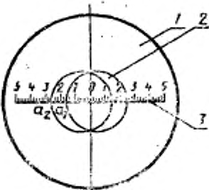
1 — поле зрения окуляра; 2 — сердцевина ОВ; 3 — шкала АТ-38 Черт. 3
