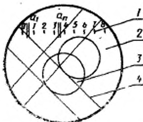
1 — шкала МОВ-1 — 15 крат; 2 — поле зрения микроскопа; 3 — сердцевина волокна; 4 — линия перекрытия Черт. 2
